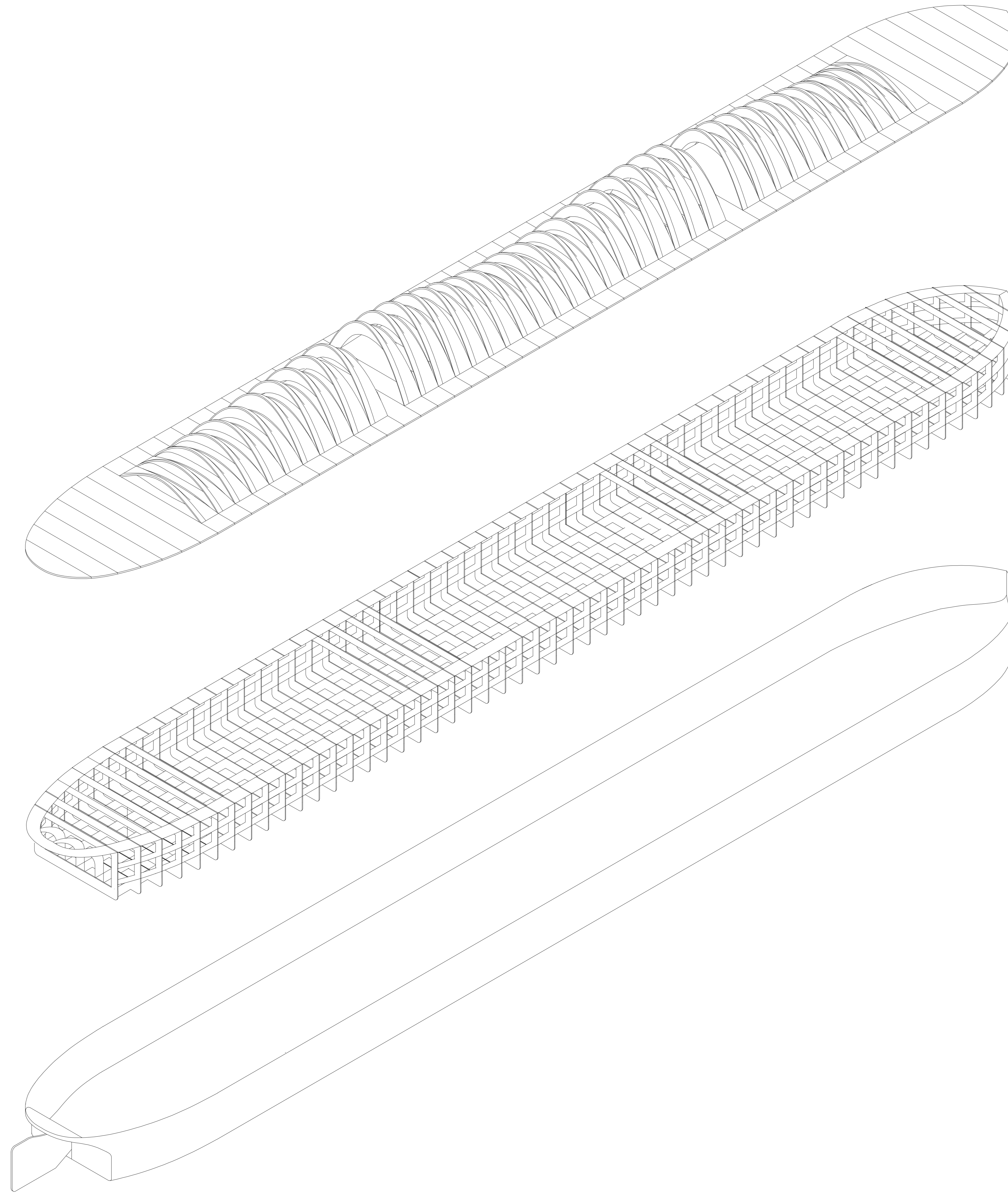
Axonometry
